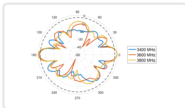
E-Plane: 3300 - 3800 MHz
