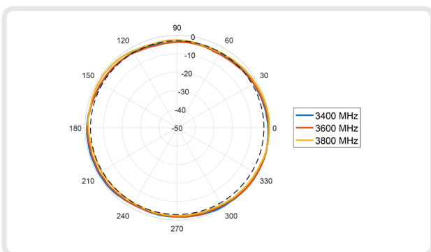
H-Plane: 3300 - 3800 MHz
