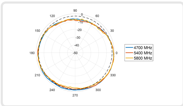
H-Plane: 4700 - 5800 MHz
