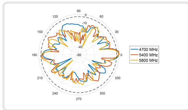
E-Plane: 4700 - 5800 MHz
