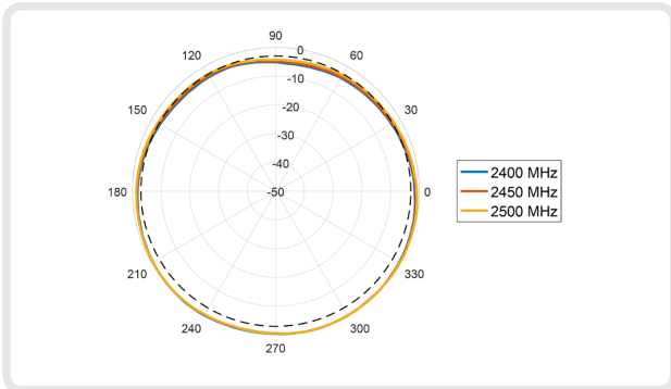
H-Plane: 2400 - 2500 MHz
