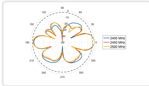
E-Plane: 2400 - 2500 MHz
