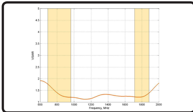
INPUT PORT VSWR:
