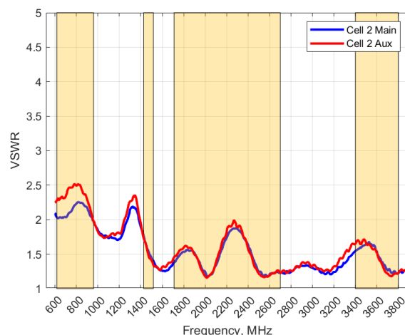
VSWR: Cell 2
